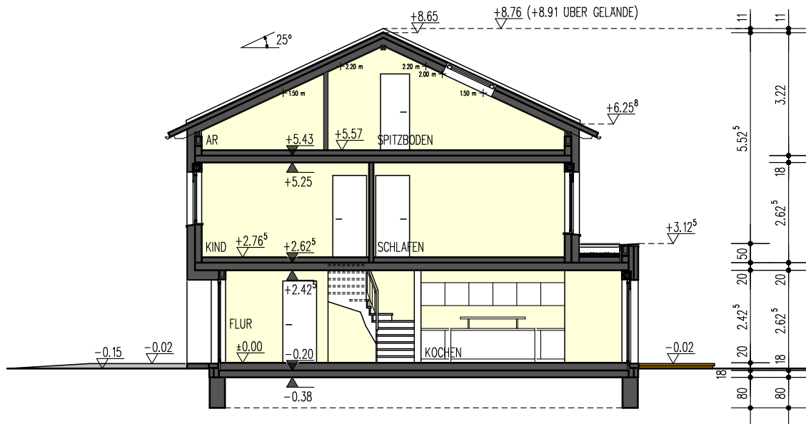
SCHNITT A-A
