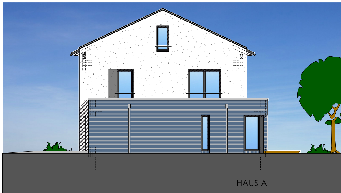
ANSICHT NORDEN
