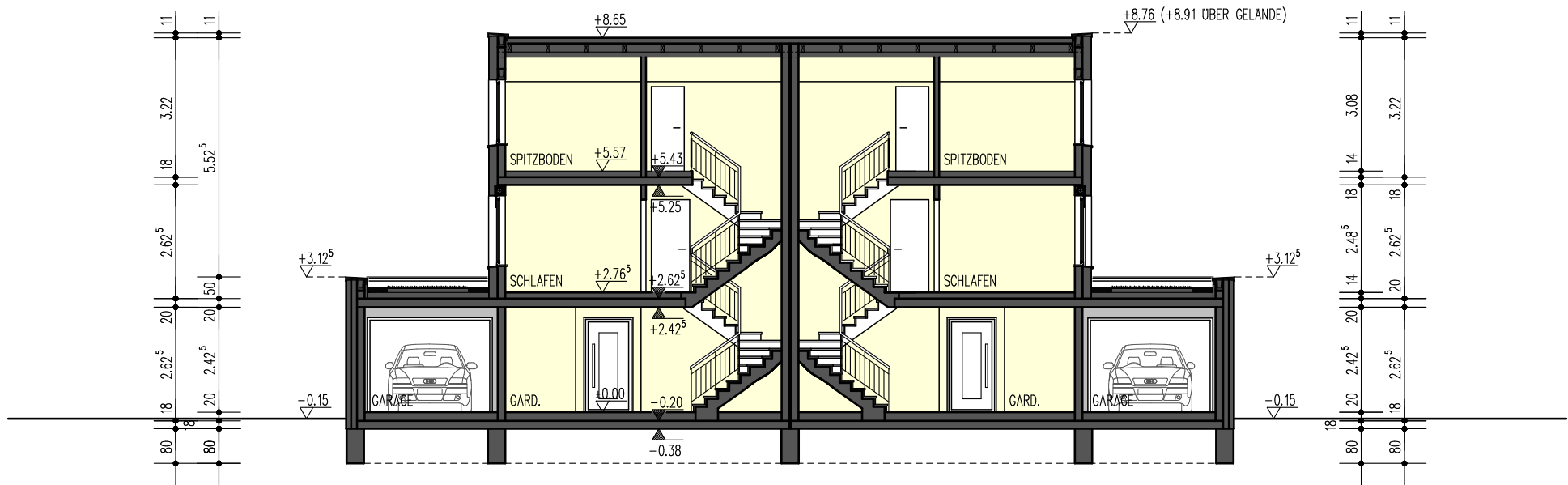
SCHNITT A-A
